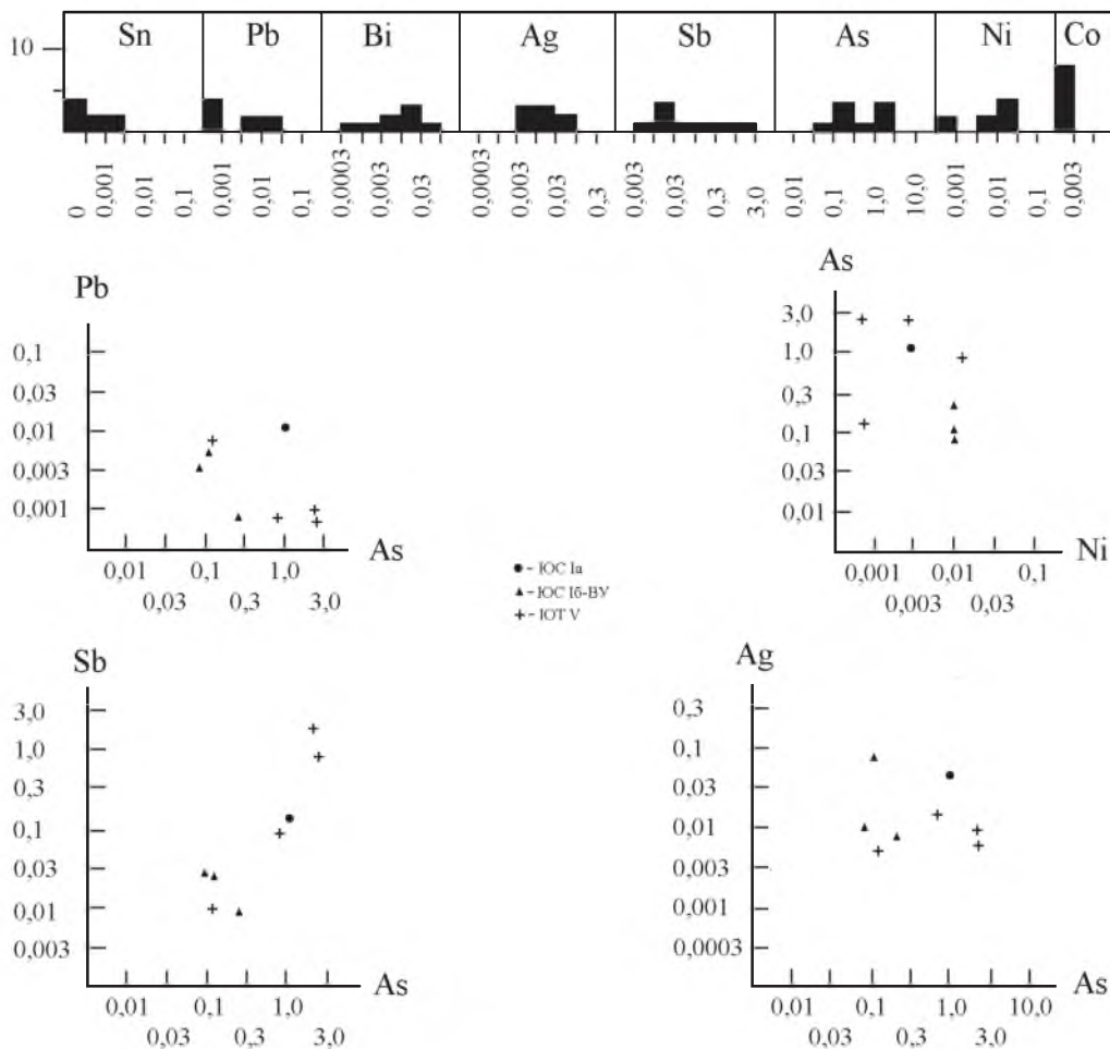
Рис. 4. Гистограммы и корреляционные графики примесей к меди могильника Шагым и случайной находки в селении Базар-Курган
